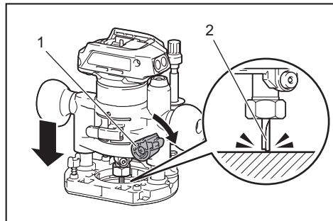
► 1. Levier de fixation 2. Embout pour affleureuse
